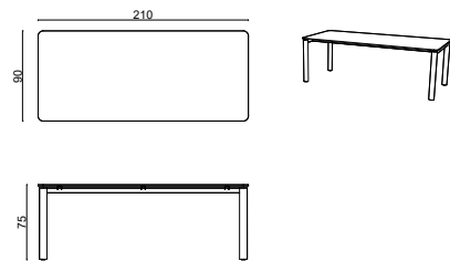
Layer Table - 90x210xh75 cm
