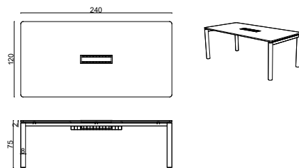
Layer Meeting Table - 120x240xh75 cm
