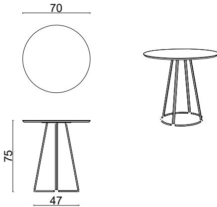
Nory Table Ø70x H 75 cm
