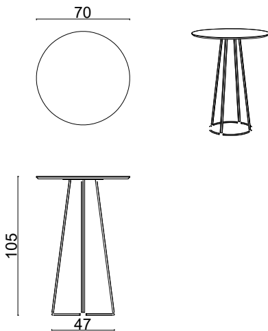
Nory Bar Table Ø70x H 105 cm
