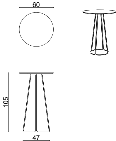
Nory Bar Table Ø60x H 105 cm
