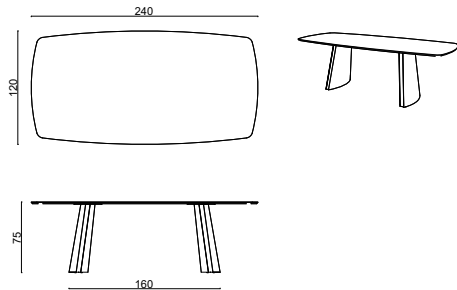
M. Allure Masa - 120x240xh75 cm
