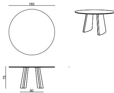
M. Allure Masa - Ø160xh75 cm
