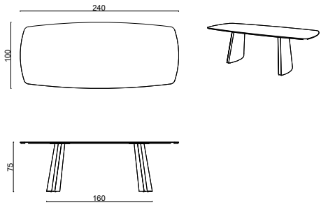
M. Allure Masa - 100x240xh75 cm
