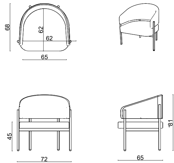
S. Hola Lounge
