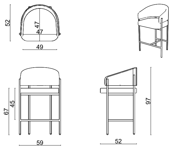
S. Hola Counter
