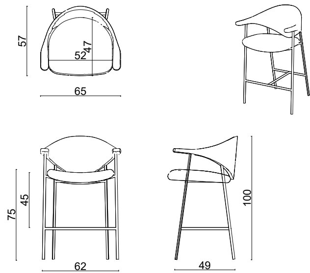
S. Trident Pipe Leg Bar
